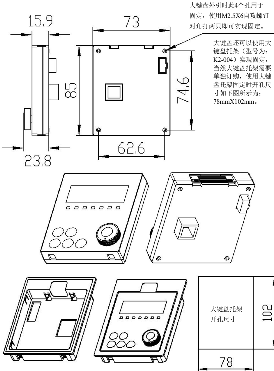
图2-6 LDE大键盘（型号为：K003-LED）/LCD中文键盘（型号为：K004-LCD）尺寸、固定方式示意图
