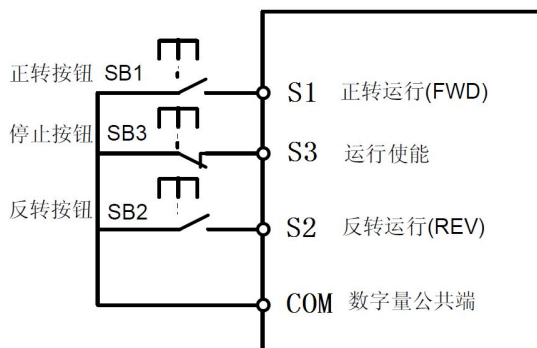
图 6-10 三线式控制模式1
