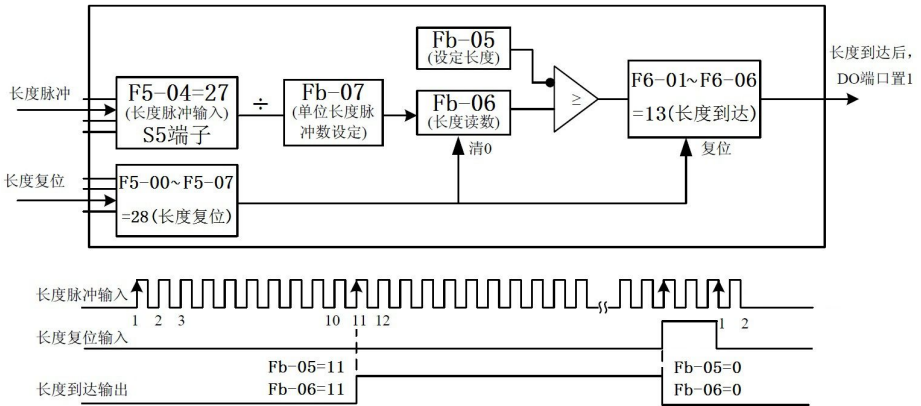
图 4-24 定长控制模式功能码设置
