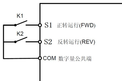
图 6-8 两线式模式1
