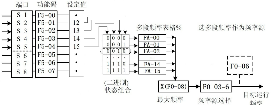
图 4-22 多段速模式的设置
