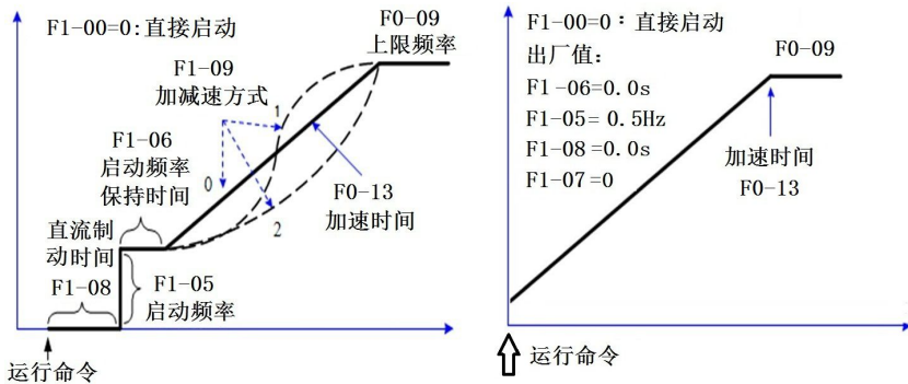
图4-7 直接启动方式
