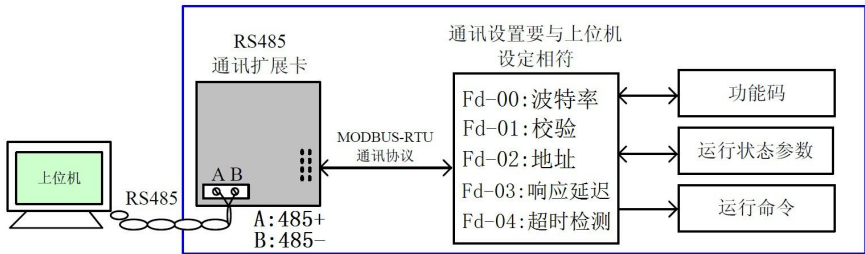
图 4-27 变频器串行通讯的使用
