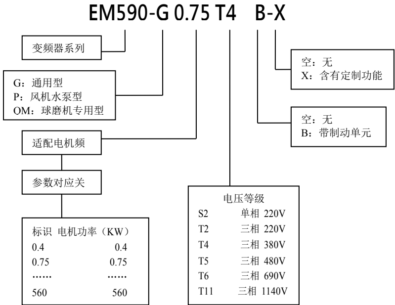
图 2-1 命名规格
