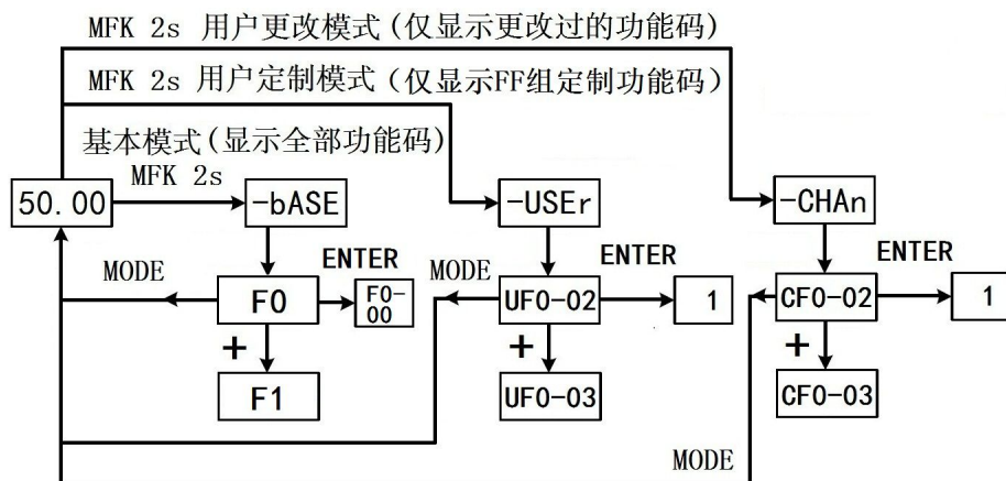
图 4-3 功能码参数快速查阅模式
