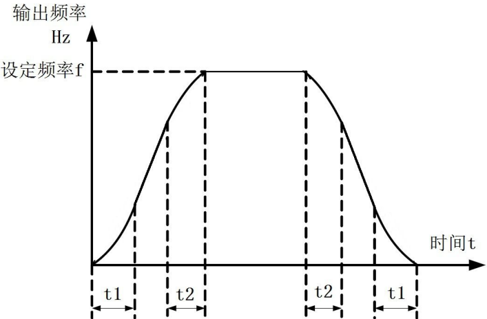
图 6-3 S曲线加减速示意图
