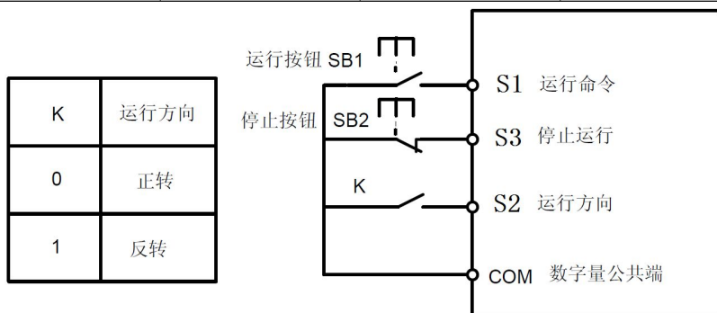
图6-11 三线式控制模式2
