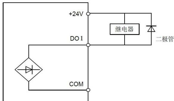
图3-10 数字输出端子接线示意图
