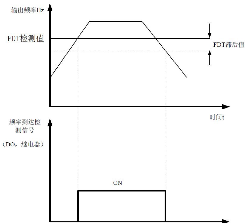
图 6-16 FDT频率检测输出示意图
