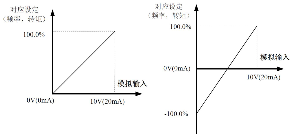
图6-12 模拟给定与设定量的对应关系
