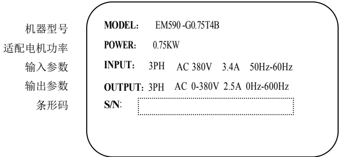
图 2-2 铭牌
