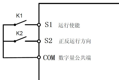
图 6-9 两线式模式2
