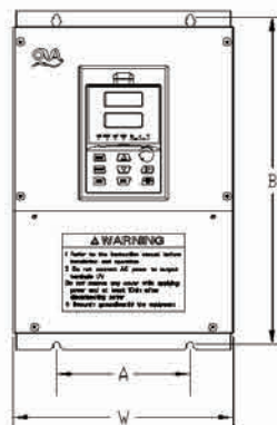
● EM600 系列金属机箱结构外型尺寸及安装尺寸示意图
