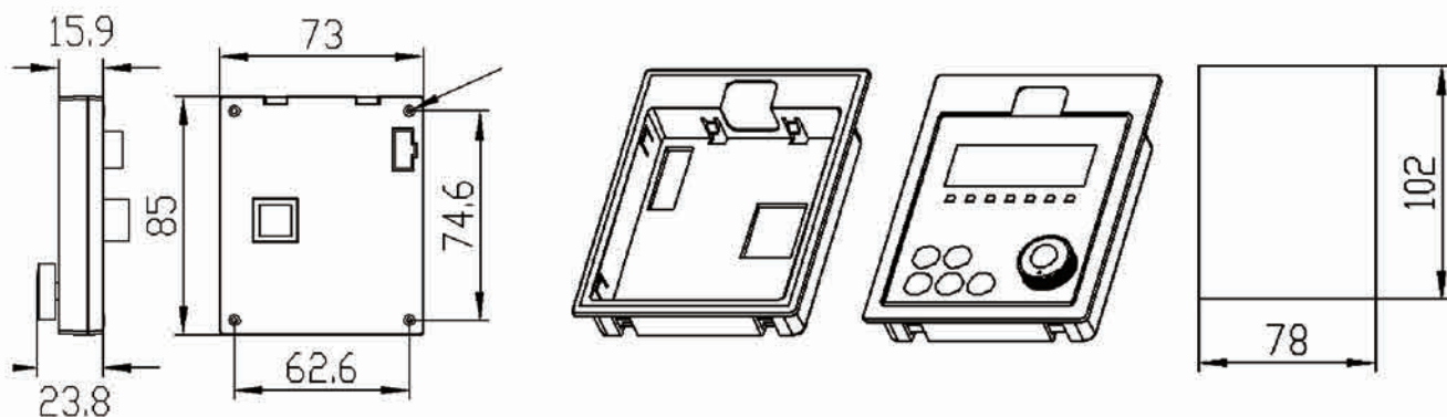
● EM590 LDE 大键盘 (型号为: K003-LED) / LCD 中文键盘 (型号为: K004-LCD) 尺寸、固定方式示意图; 外引大键盘开孔尺寸为 78X102
