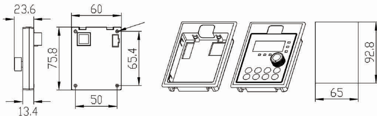
● EM590 小键盘 (型号为: K002-LED) 尺寸、固定方式示意图; 外引小键盘开孔尺寸为 65X92.8
