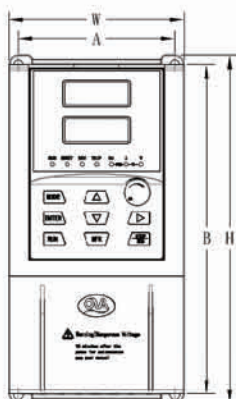
● EM600 系列塑胶机箱结构外型尺寸及安装尺寸示意图
