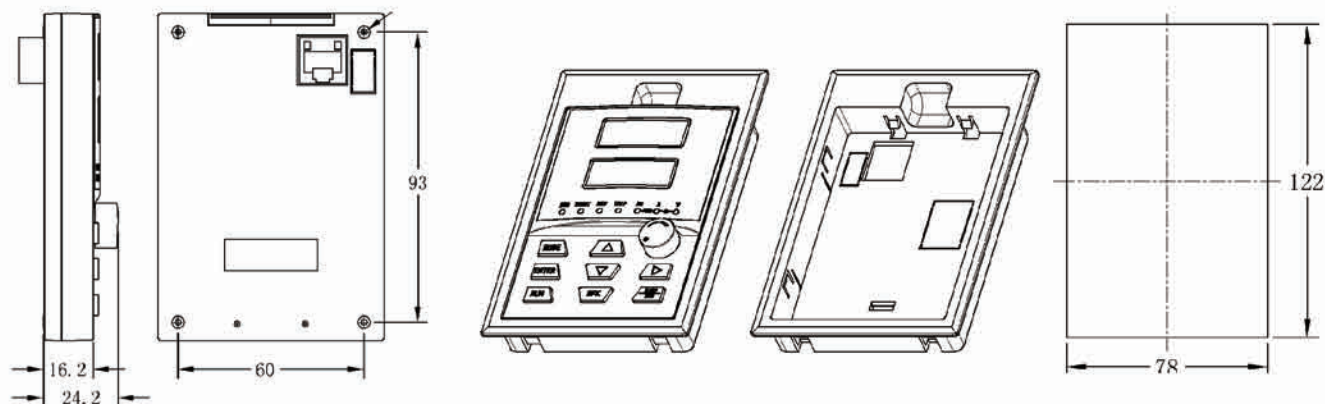
● EM600 键盘 (型号为: MON1012) 尺寸、固定方式示意图; 外引键盘开孔尺寸为 78X122
