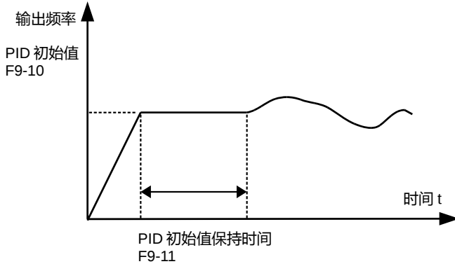
图6-19 PID 预置频率功能
