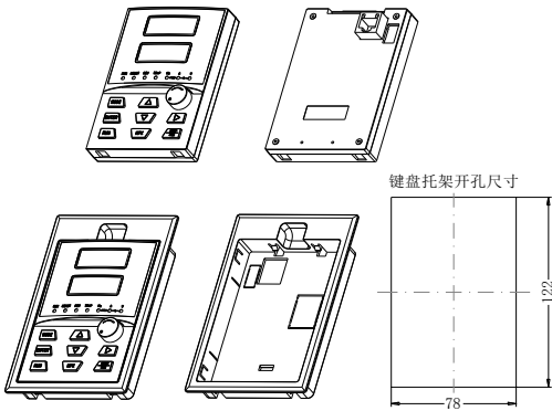
图2-6 双行LDE键盘（型号为：K6902-LED-2） LCD中文键盘（型号为：K004-LCD）尺寸、固定方式示意图
