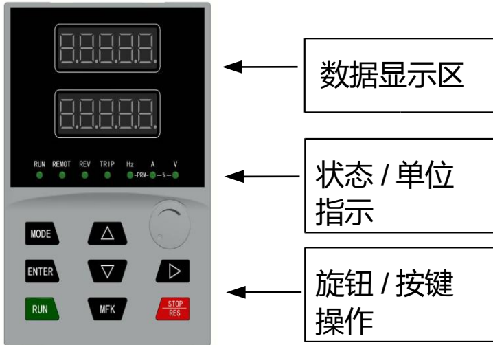
图4-1 操作键盘示意图
