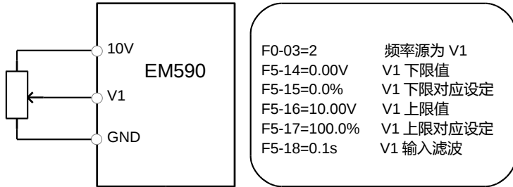
图 4-15 V1电压型输入给定频率功能码设置
