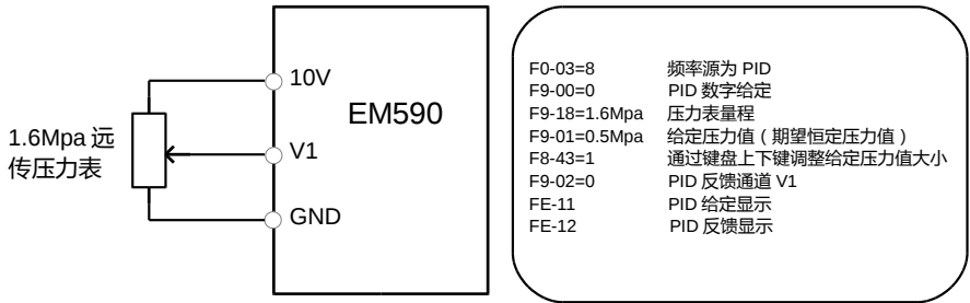
图 4-18 恒压供水应用
