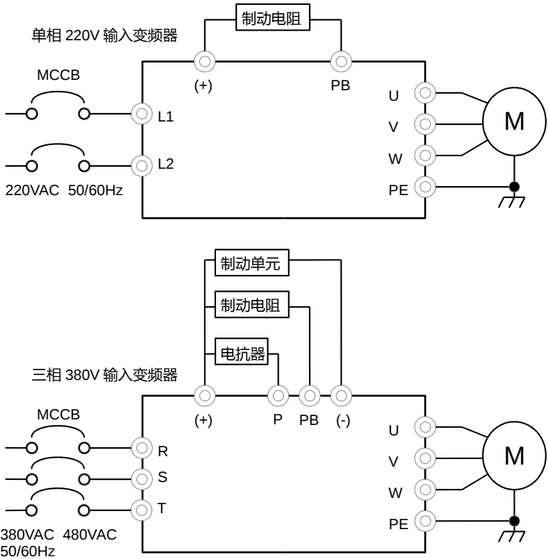
变频器主路接线方式
