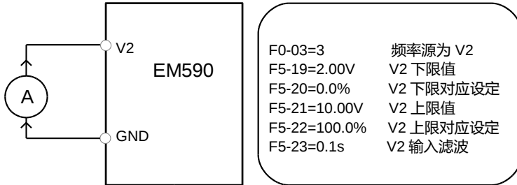
图 4-16 V2电流型输入给定频率功能码设置
