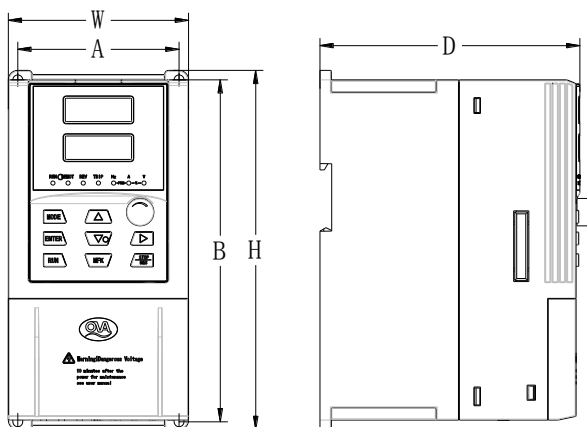
图 2-3 EM590N系列塑胶机箱结构外型尺寸及安装尺寸示意图
