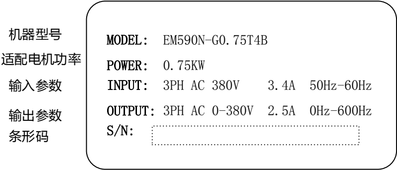
图 2-2 铭牌
