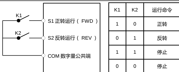
图 6-8 两线式模式1
