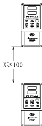
上下安装示意图
