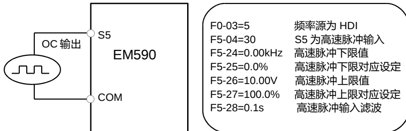
图 4-17 脉冲给定频率功能码设置
