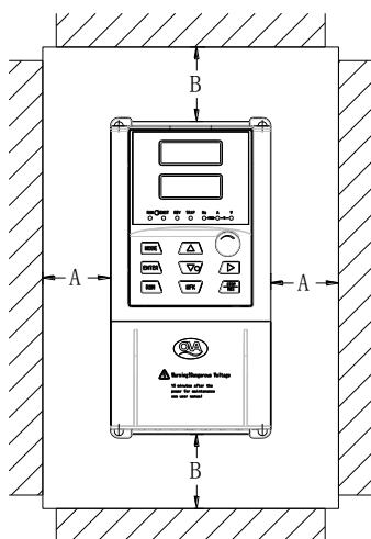
单体安装示意图
