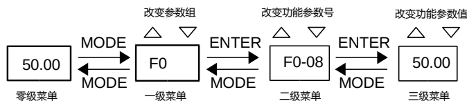
图4-2 三级菜单操作流程图
