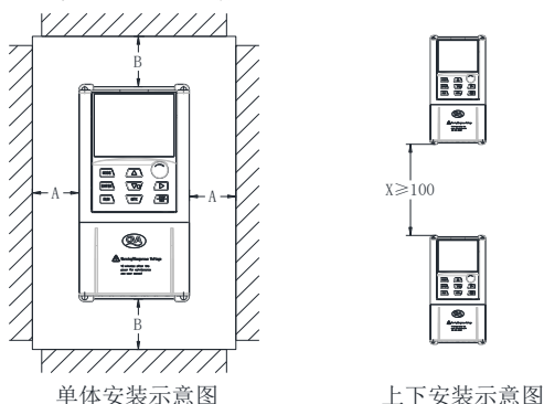
图3-1变频器安装示意图
