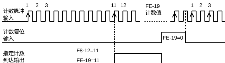
图6-14 指定计数值给定示意图
