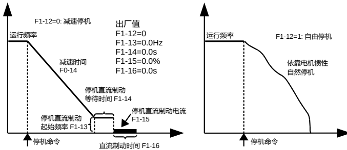
图 4-10 停机方式
