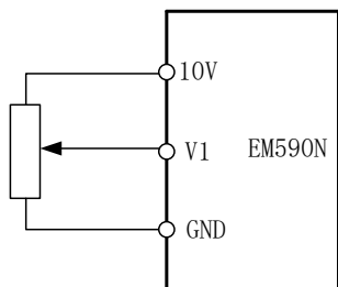
图 4-15 V1电压型输入给定频率功能码设置
