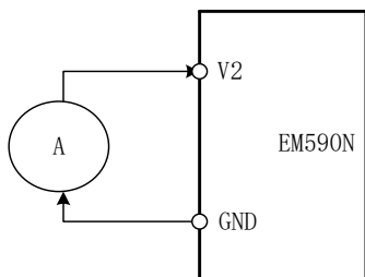
图 4-16 V2电流型输入给定频率功能码设置
