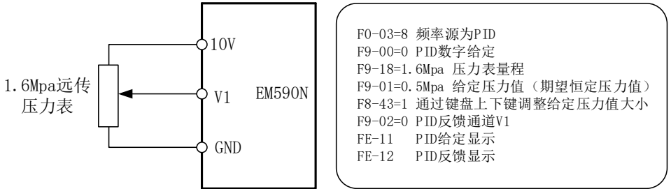
图 4-18 恒压供水应用
