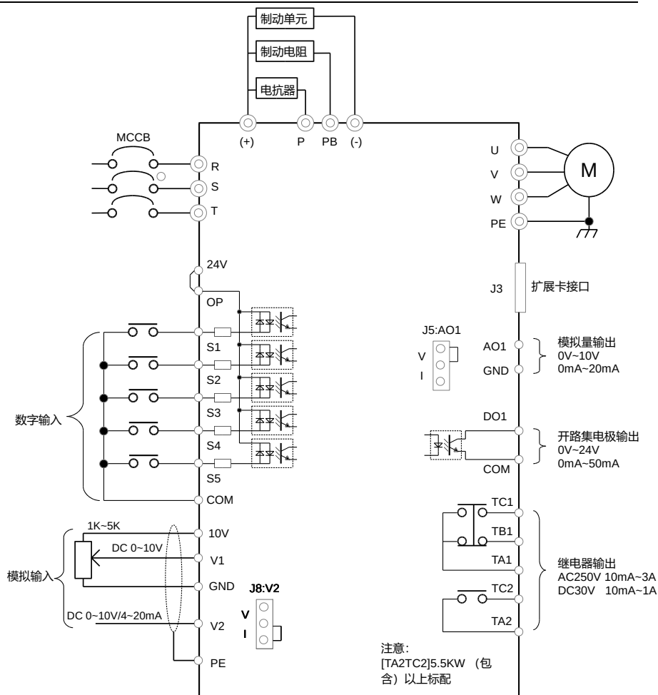
图3-4 三相380V主回路和控制回路接线方图
