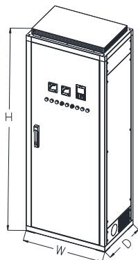
图 2-5 EM590N系列柜机机箱结构外型尺寸示意
