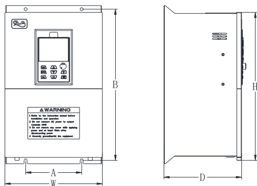
图 2-4 EM590N系列金属机箱结构外型尺寸及安装尺寸示意图
