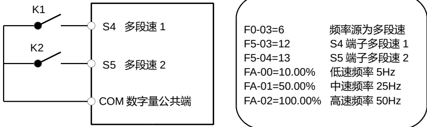
图 4-19 多段速模式的设置
