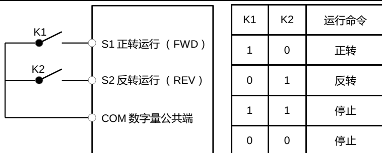
图 6-8 两线式模式1
