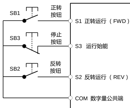
图 6-10 三线式控制模式1
