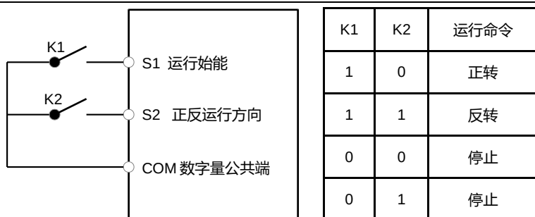
图 6-9 两线式模式2
