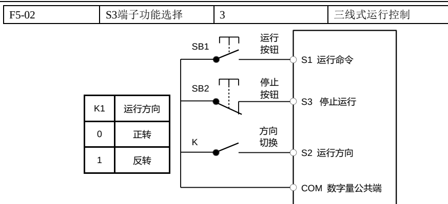
图6-11 三线式控制模式2
