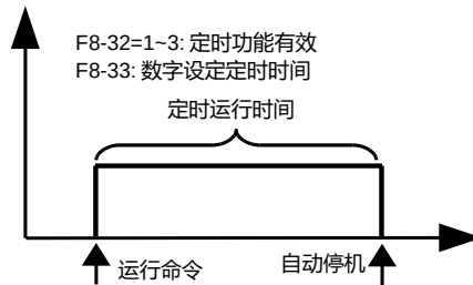
图4-11 定时停机功能
