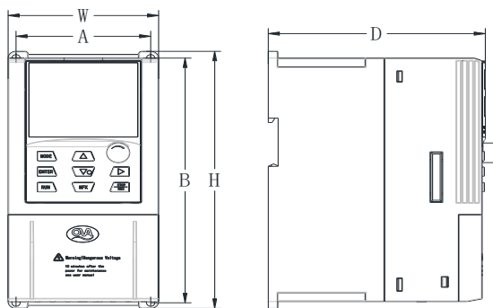
图 2-3 EM590N系列塑胶机箱结构外型尺寸及安装尺寸示意图
