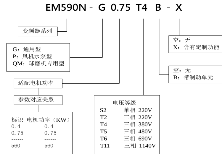
图 2-1 命名规格
