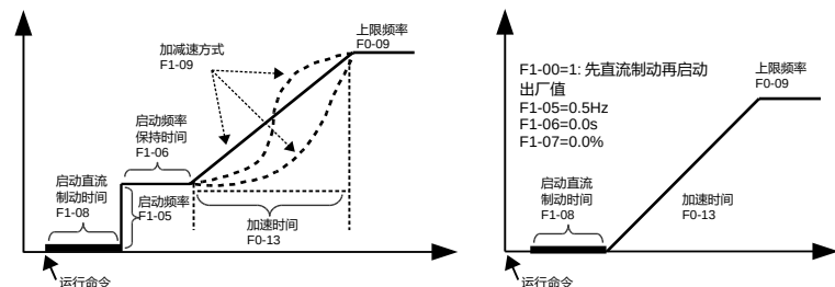
图4-8 先直流制动再启动
