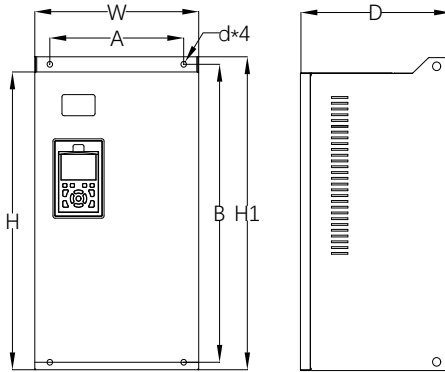
图 2-3：205~212 钣金机箱代码尺寸示意图
