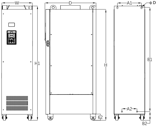
图 2-4：213~215 钣金机箱代码尺寸示意图
