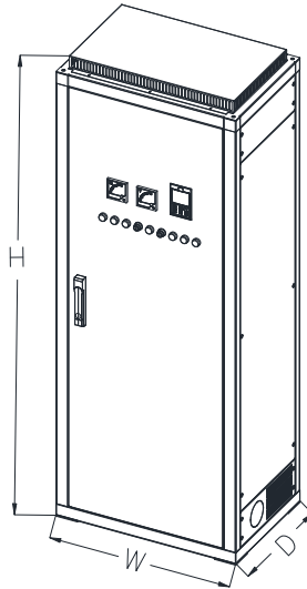
图 2-5：913~925 钣金机箱代码尺寸示意图
