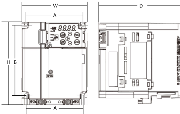
图 2-2: 201~204 机箱代码尺寸示意图
