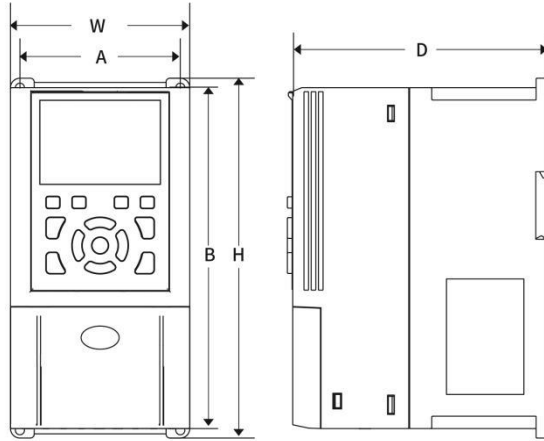
图 2-1: 101~102 机箱代码尺寸示意图
